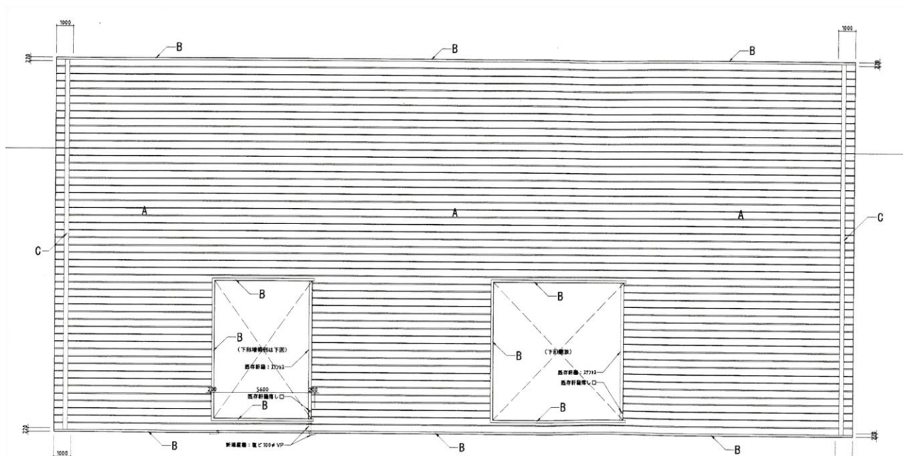
施設屋根部平面図
