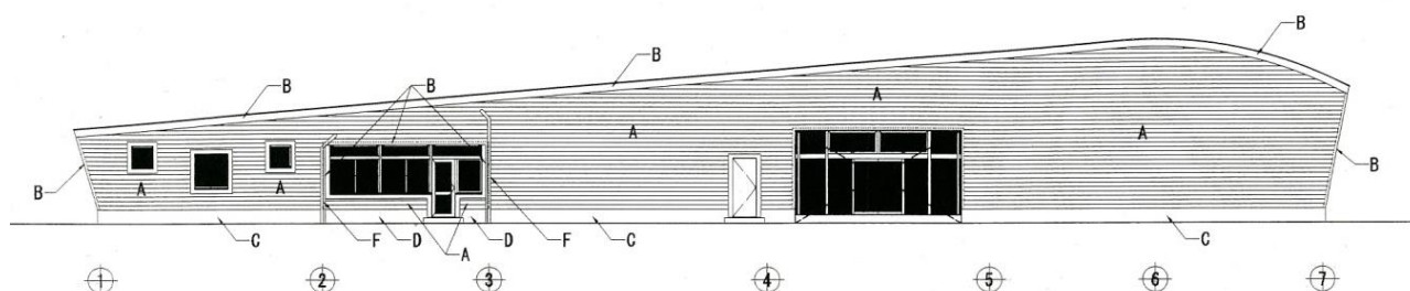
ガイダンス施設南側側面図
