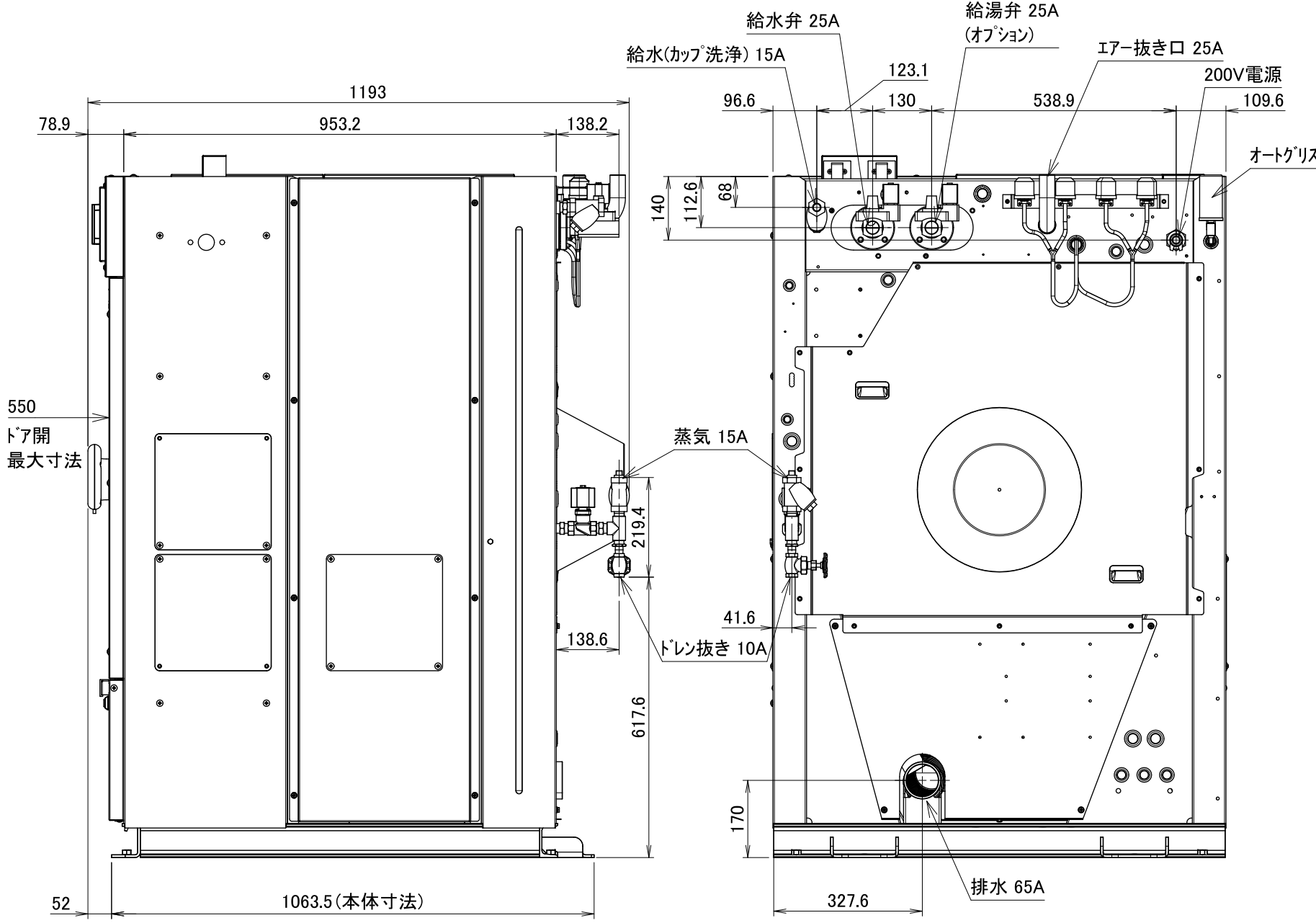
WN230外観図
