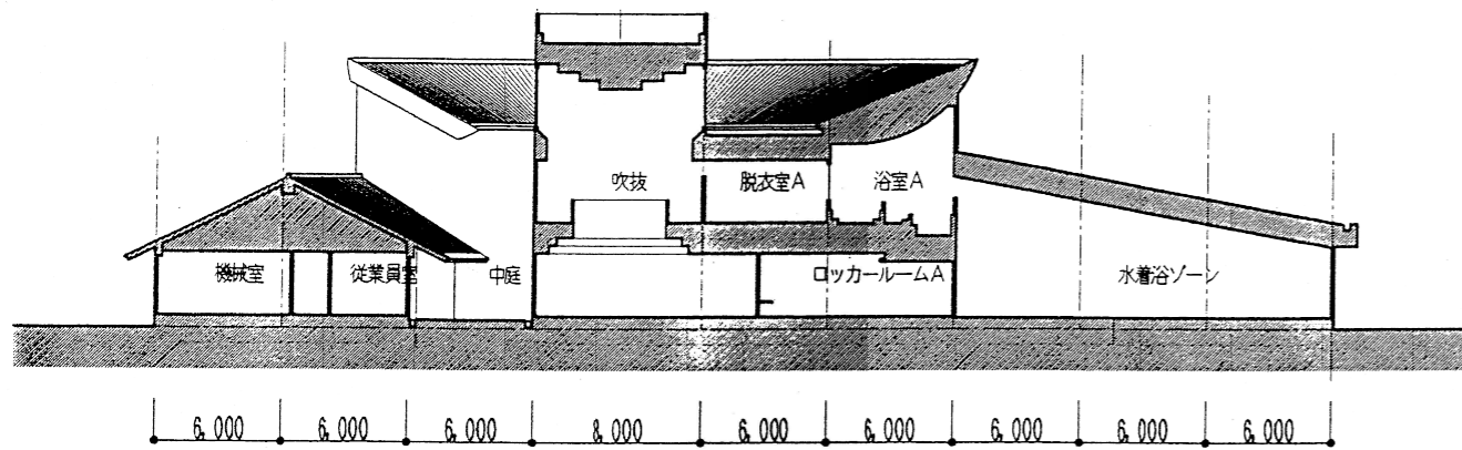
A A断面図
