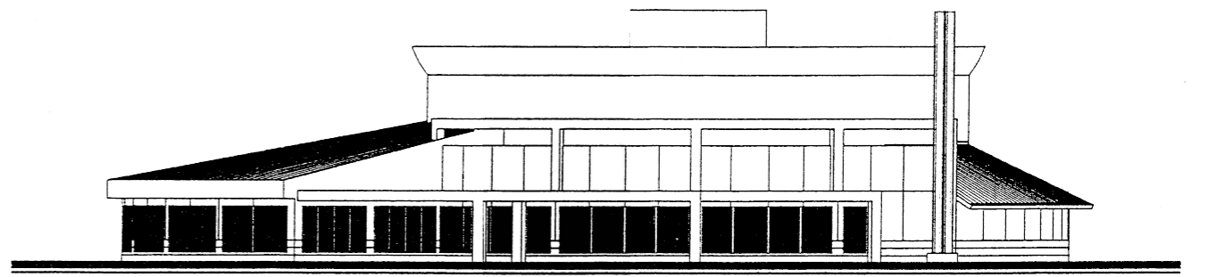
北 立面図
