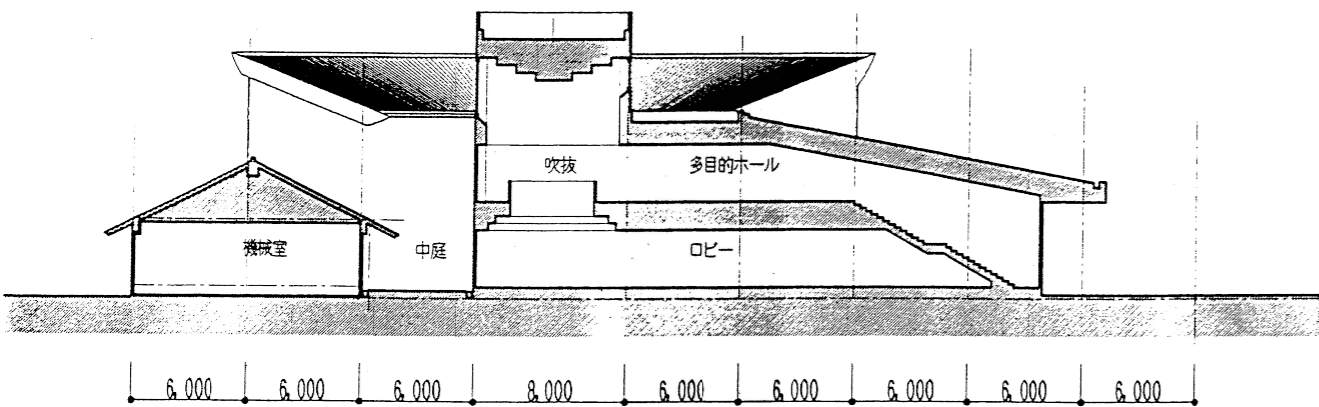
C C断面図
