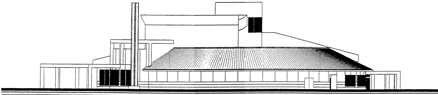
西 立面図
