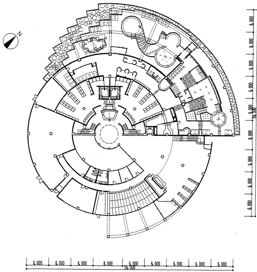
1階平面図
