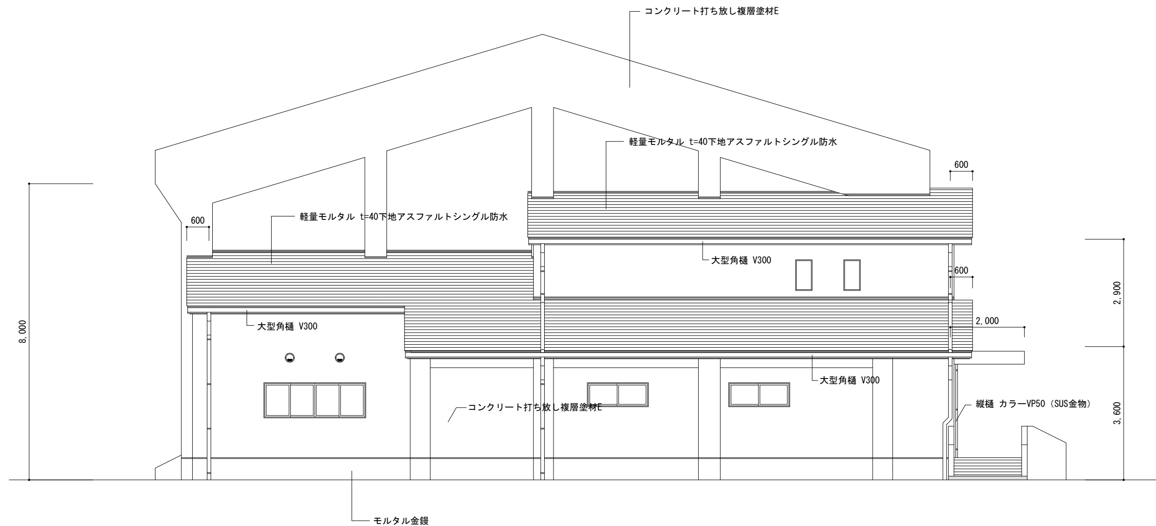
北立面図 S=1/100
