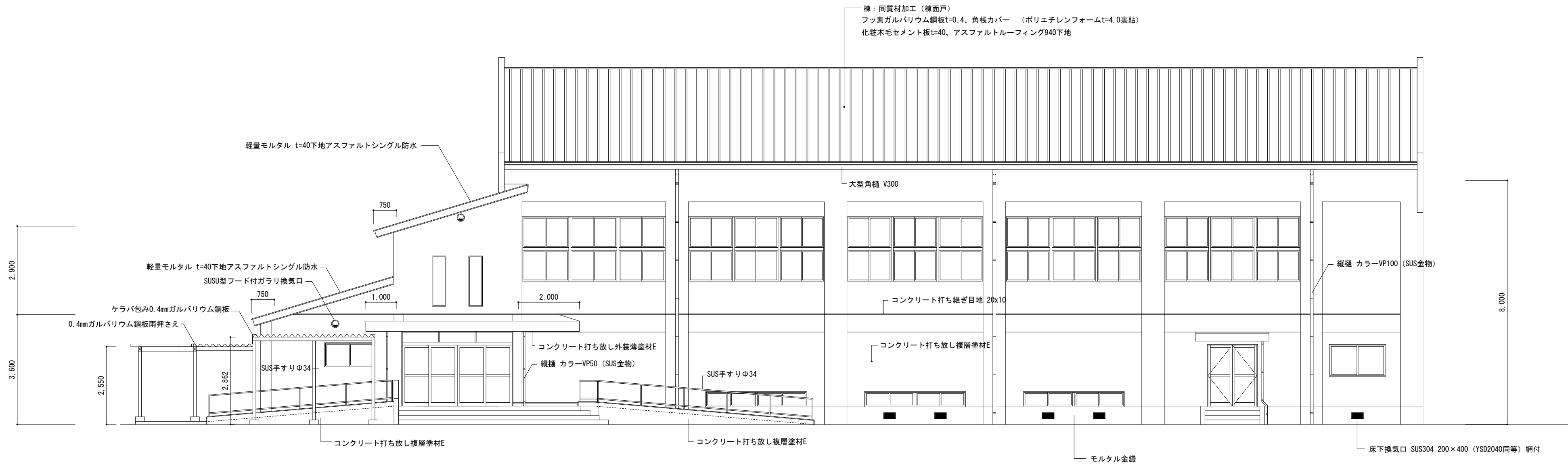
西立面図 S=1/100
