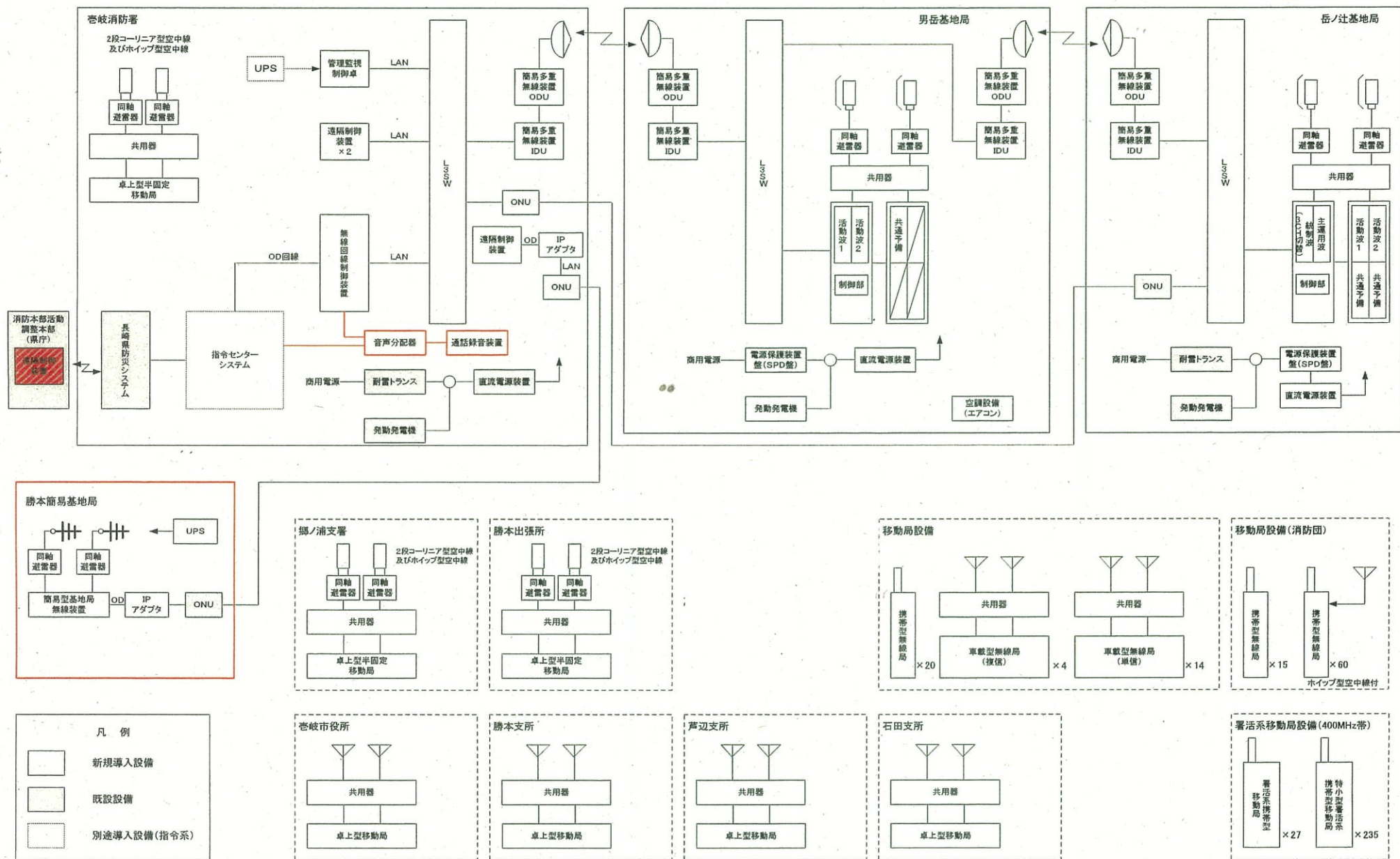
図1 梶崎市消防本部 消防救急デジタル無線設備 システム構成図
