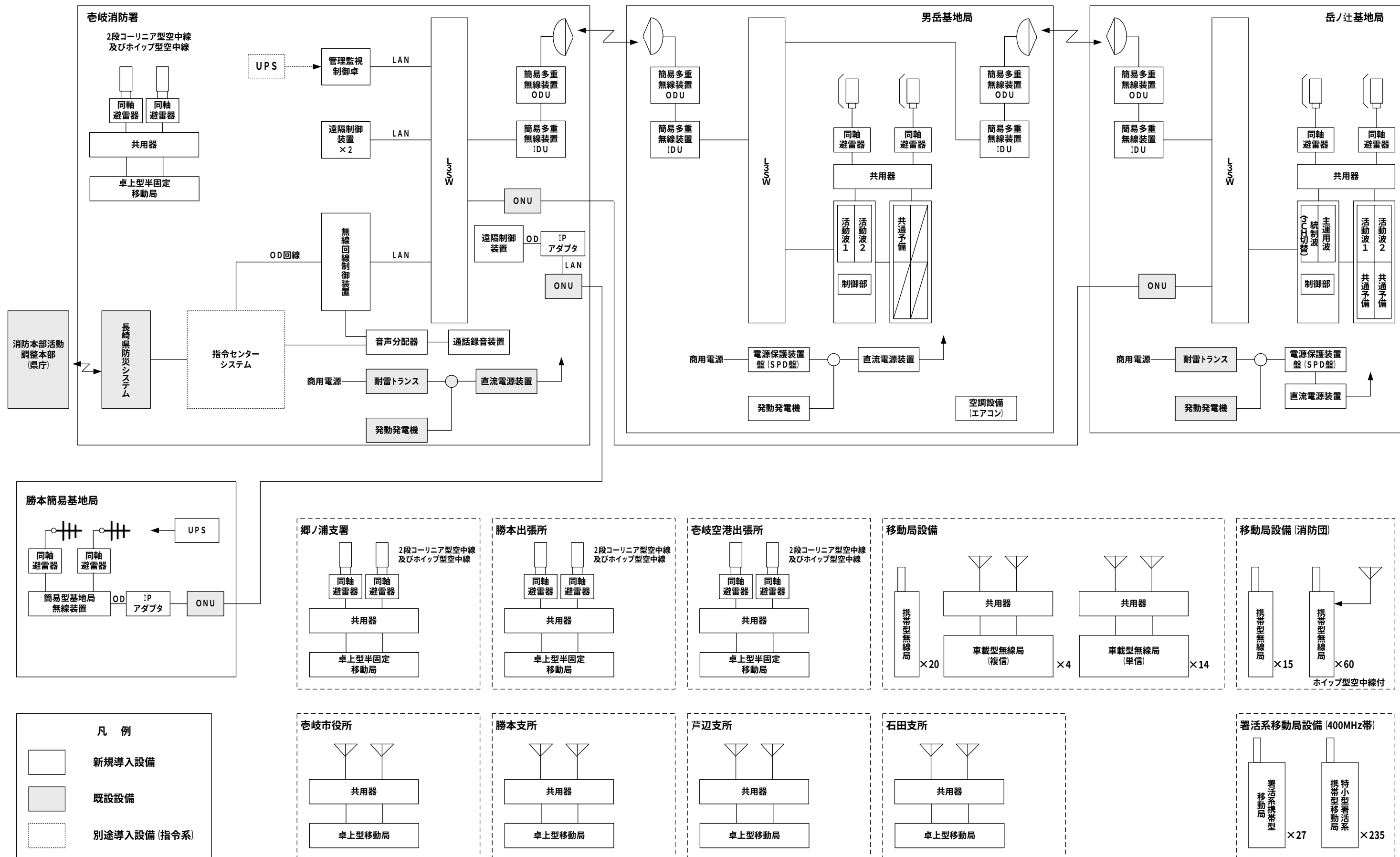
図1 壱岐市消防本部 消防救急デジタル無線設備 システム構成図
