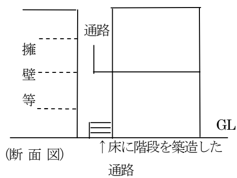
例図5（共同住宅）
