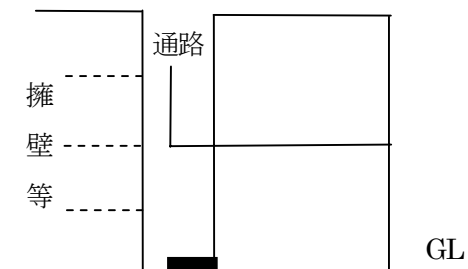
例図4（1階長屋）
