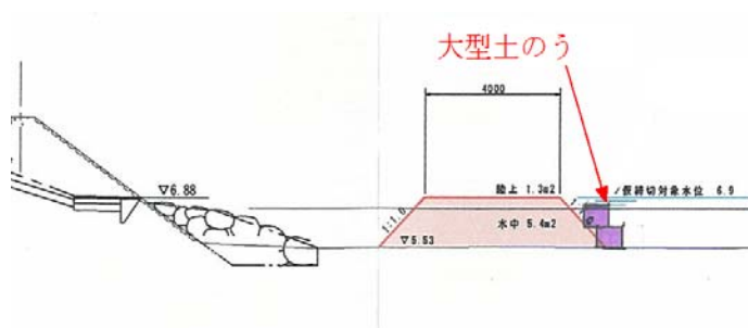
標準断面図
