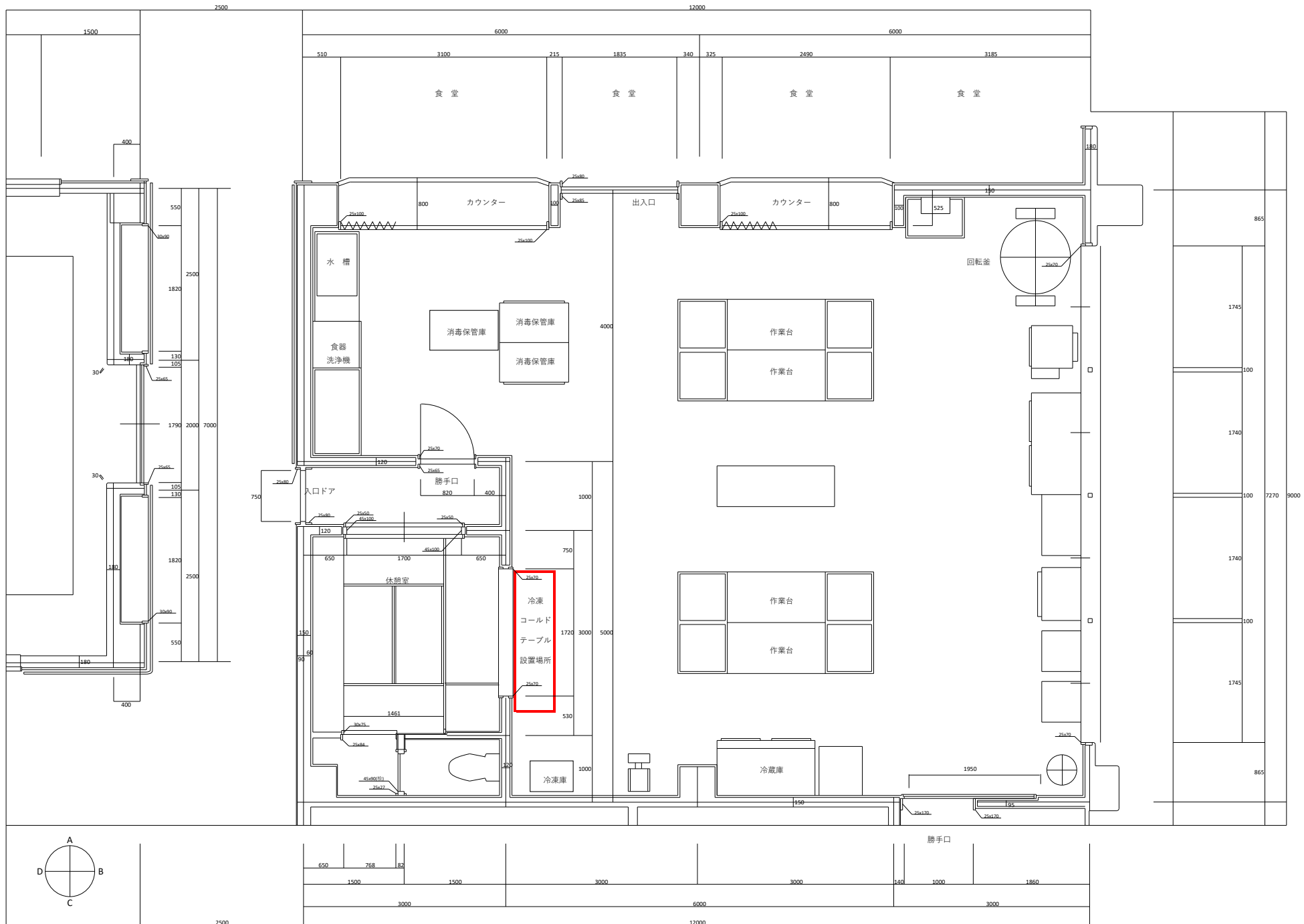
調理室 平面図 S=1/30
